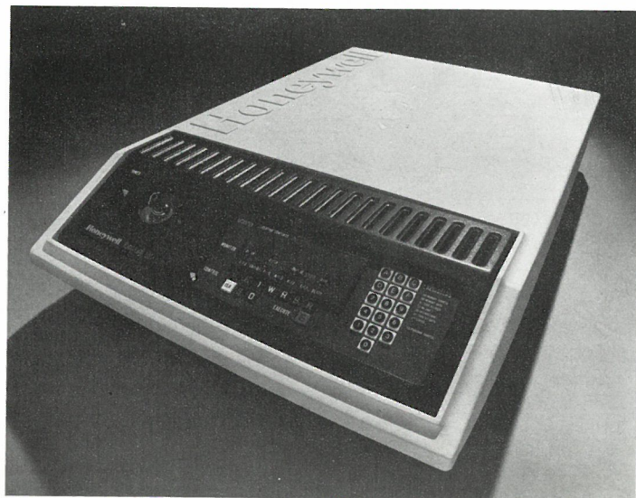
Un Honeywell livello 6 nella versione Table-Top. Si tratta di un Modello 43 con 256 K bytes di memoria, governo per 4 dischi, governo per 4 periferiche ed otto linee. Assai interessanti sono le ridotte proporzioni del sistema: altezza cm 14, lunghezza cm 47, larghezza cm 49.
